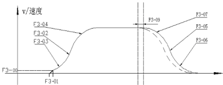
图6-3 速度曲线图
