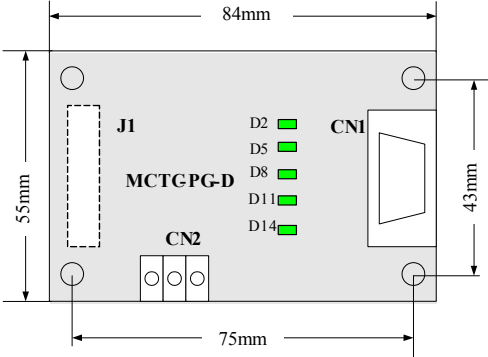
图3-8 MCTC-PG-D尺寸图
