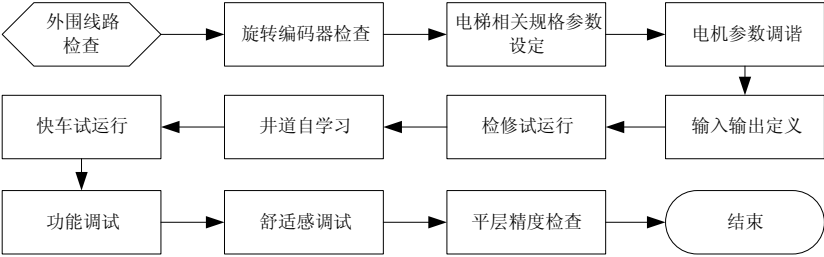
图7-1 调试流程
