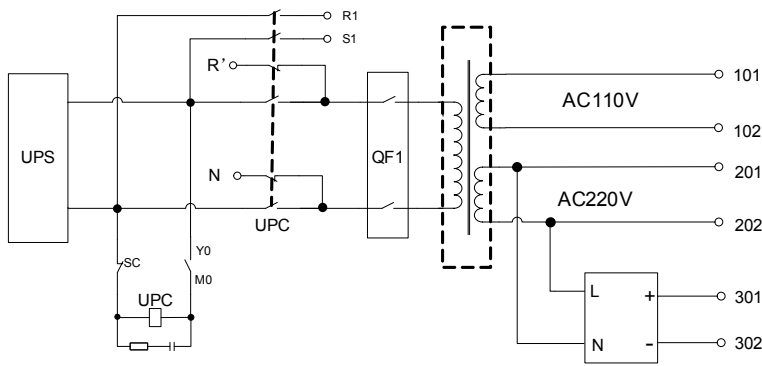
图7-4 应急电源回路参考图
