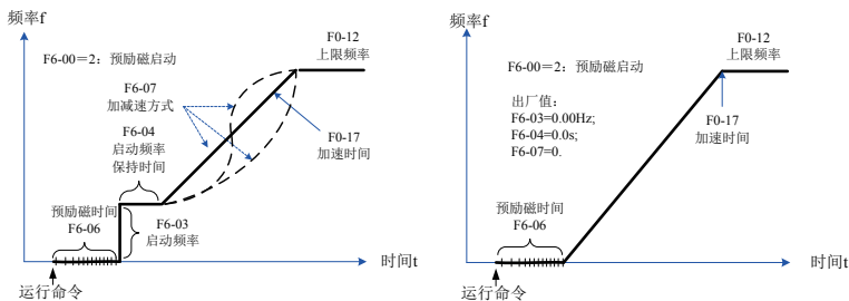
图 4-11 预励磁启动方式
