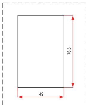
图 D-3 MD310-KEY1 外引键盘安装尺寸图 (单位: mm)
