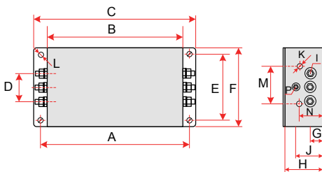
图 7-3 共模滤波器 DL-25EBK5/DL-35EBK5/ DL-50EBK5 尺寸图
