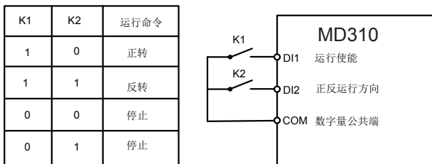
图 6-13 两线式模式 2
