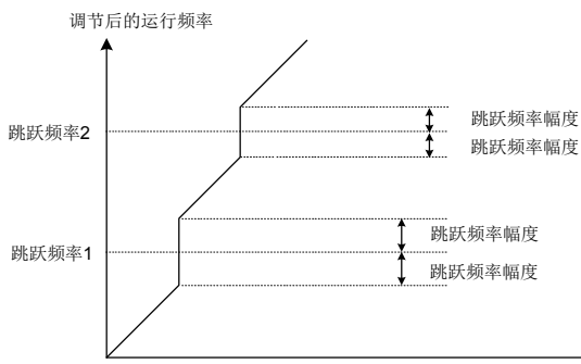
图 6-24 加减速过程中跳跃频率有效示意图
