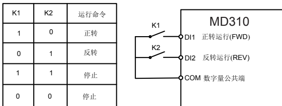
图 6-12 两线式模式 1
