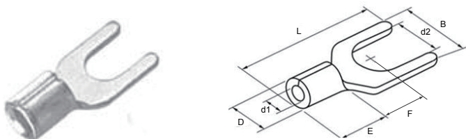
图 3-12 TNS 系列叉形线耳外观及尺寸图（【注】）
