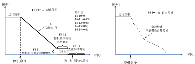
图 4-12 停机模式
