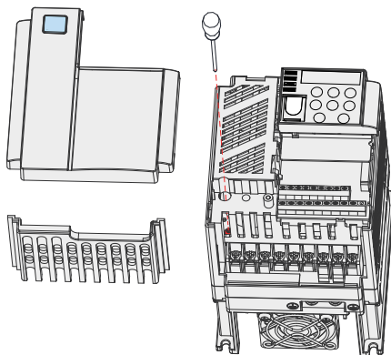
图 7-10 MD310T0.4B、MD310T0.7B、MD310T1.5B、MD310T2.2.2B 压敏电阻（VAR）和安规电容共同对 PE 连接的螺钉位置示意图
