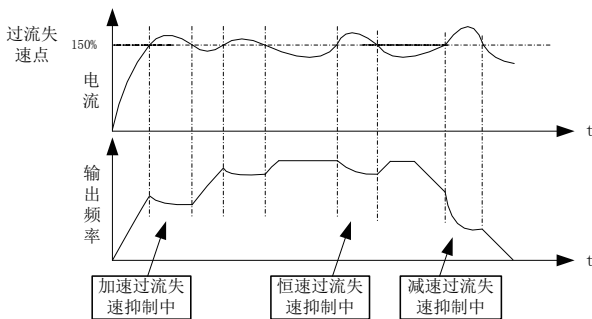
图 6-9 过流失速动作示意图
